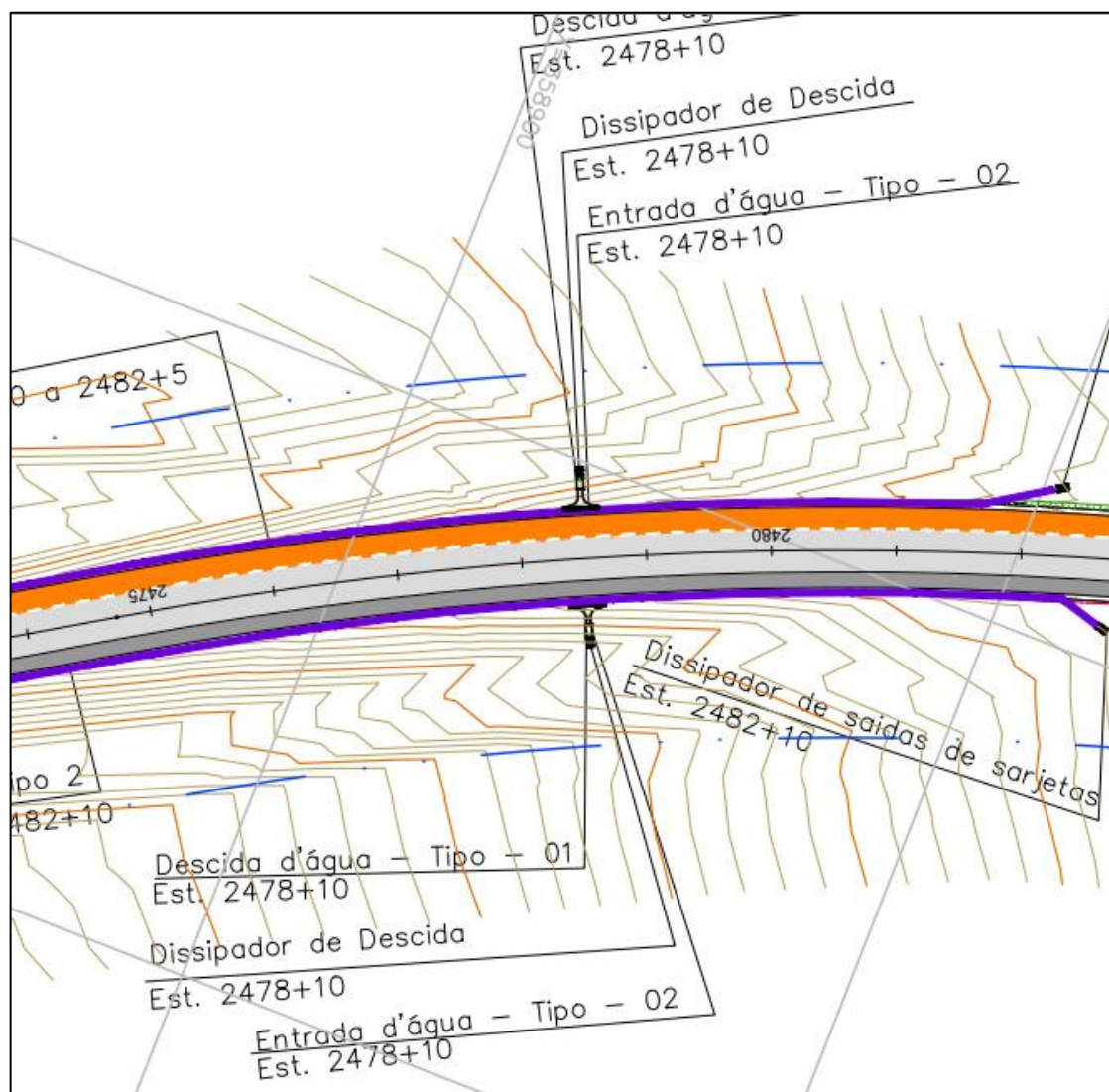
Figura 4 – Indicação de elementos de drenagem
