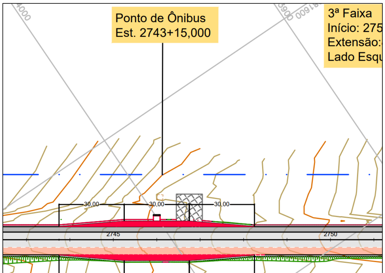
Figura 1 - Etiqueta localizada na estaca 2746+2,50, indicando estaca 2743+15,00
