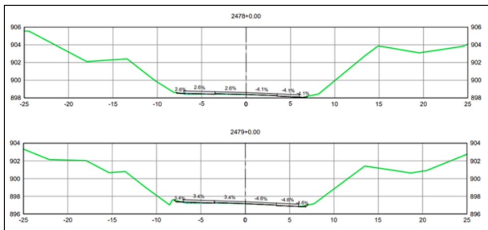
Figura 5 - Seções do projeto de terraplenagem
