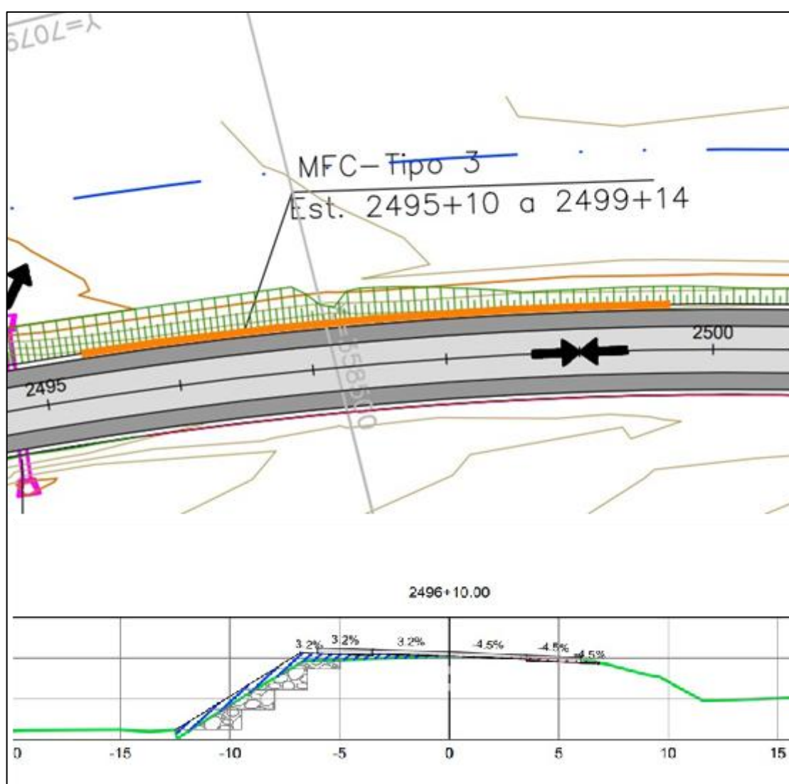
Figura 3 - Indicação de meio-fio do lado alto da elevação da curva
